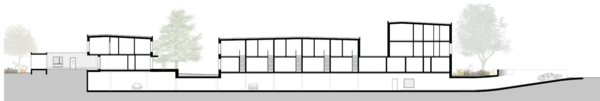
coupe F-F
